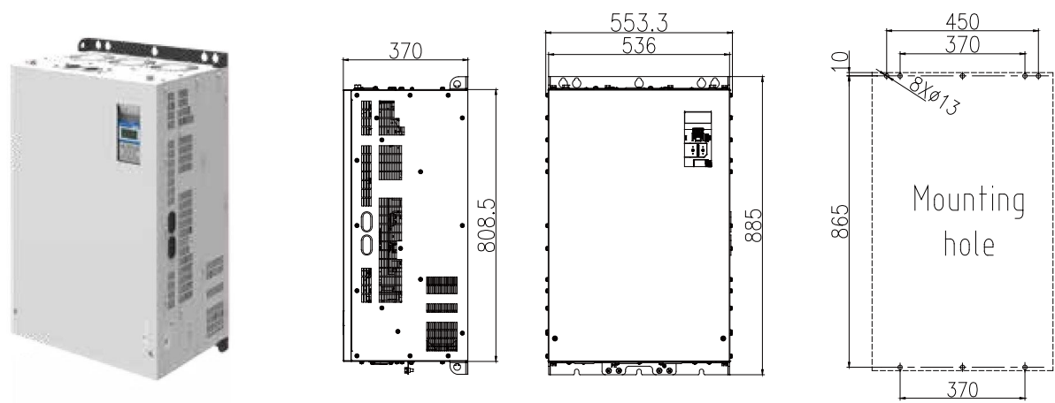
◆B7(160kW ~ 250kW)
