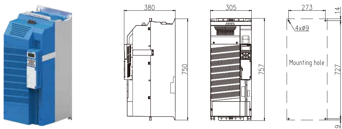
◆B7(160kW ~ 250kW)
